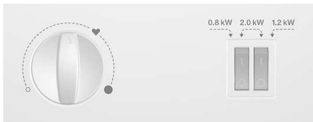
Рисунок 2. Панель управления водонагревателя
