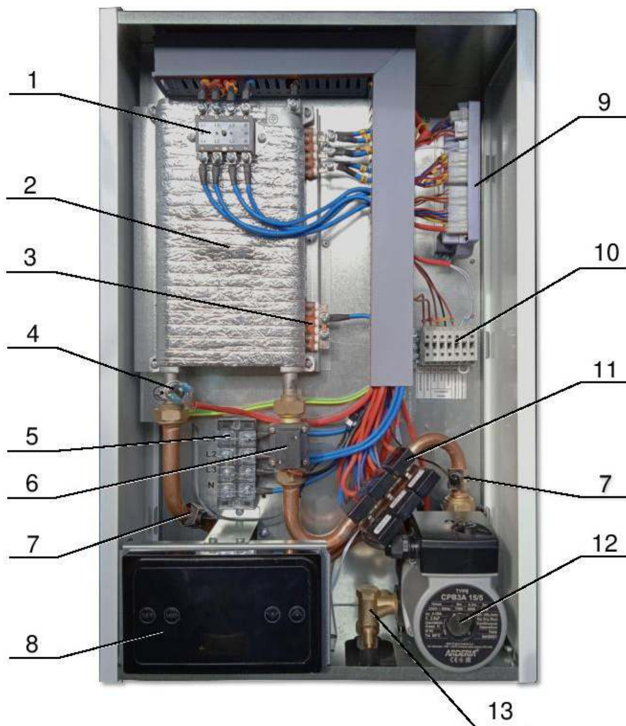
Рис. 1 Общий вид
