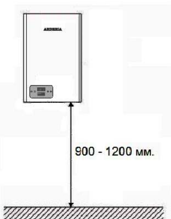
Рис. 10 Монтажные расстояния
