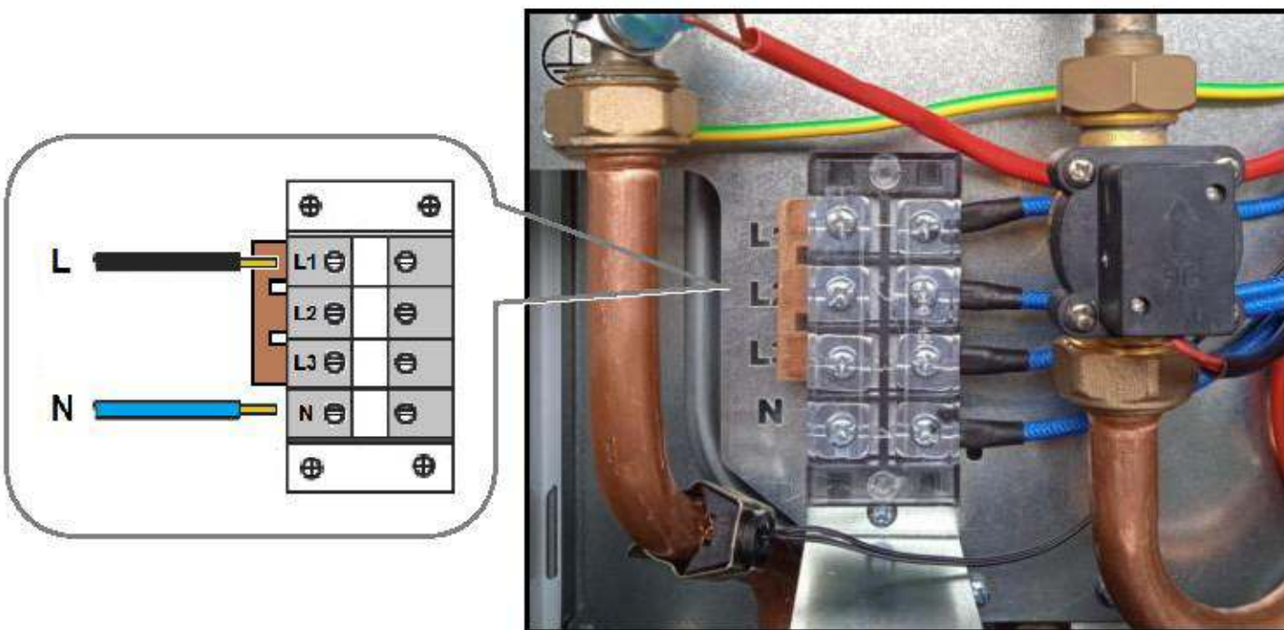
Рис. 15 Однофазное подключение
