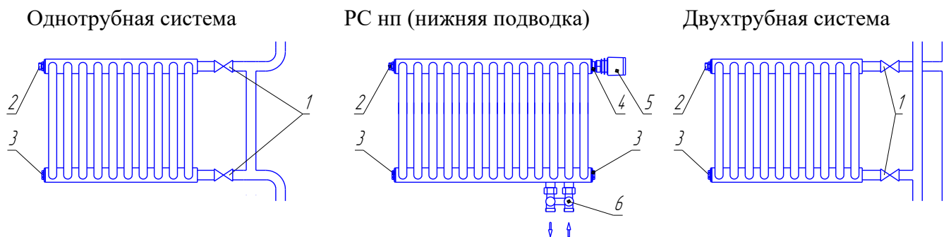
1. Вентиль. 2. Кран Маевского-воздухоотводчик. 3. Пробка глухая. 4. Клапан терморегулятора. 5. Термостатический элемент. 6. Запорно-присоединительный клапан нижнего подключения.
