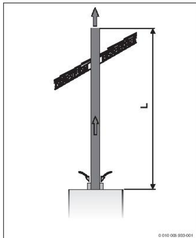
Рис. 5 Вертикальный отвод дымовых газов B_{22}
