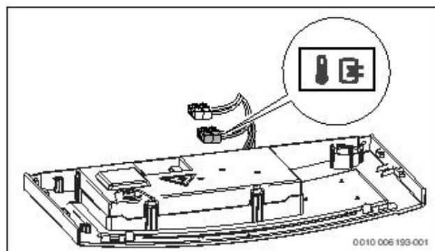
Рис. 23 Подключение датчика температуры бака-водонагревателя
