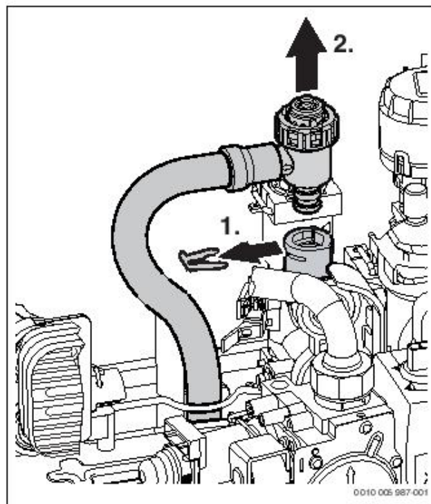
Рис. 35 Демонтаж предохранительного клапана (отопительного контура)
