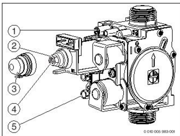
Рис. 32 Газовая арматура
