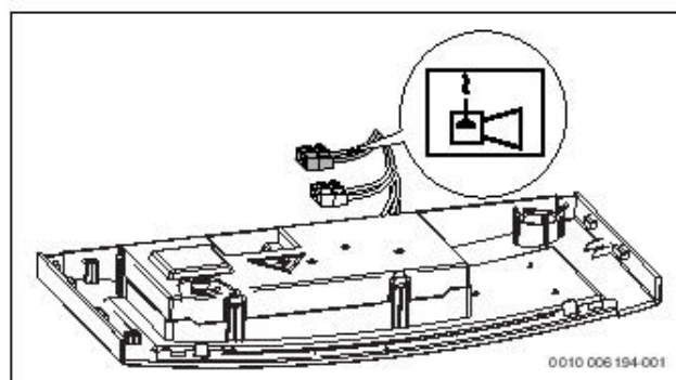
Рис. 24 Подключение сигнала тревоги
