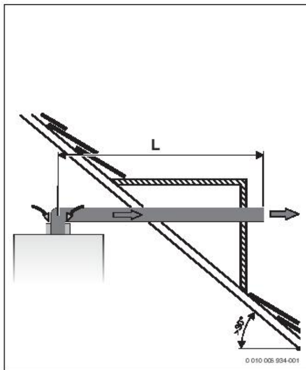
Рис. 4 Горизонтальный отвод дымовых газов B_{22}
