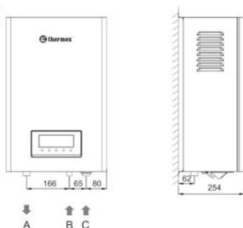
Рис. 7. Присоединительные размеры
