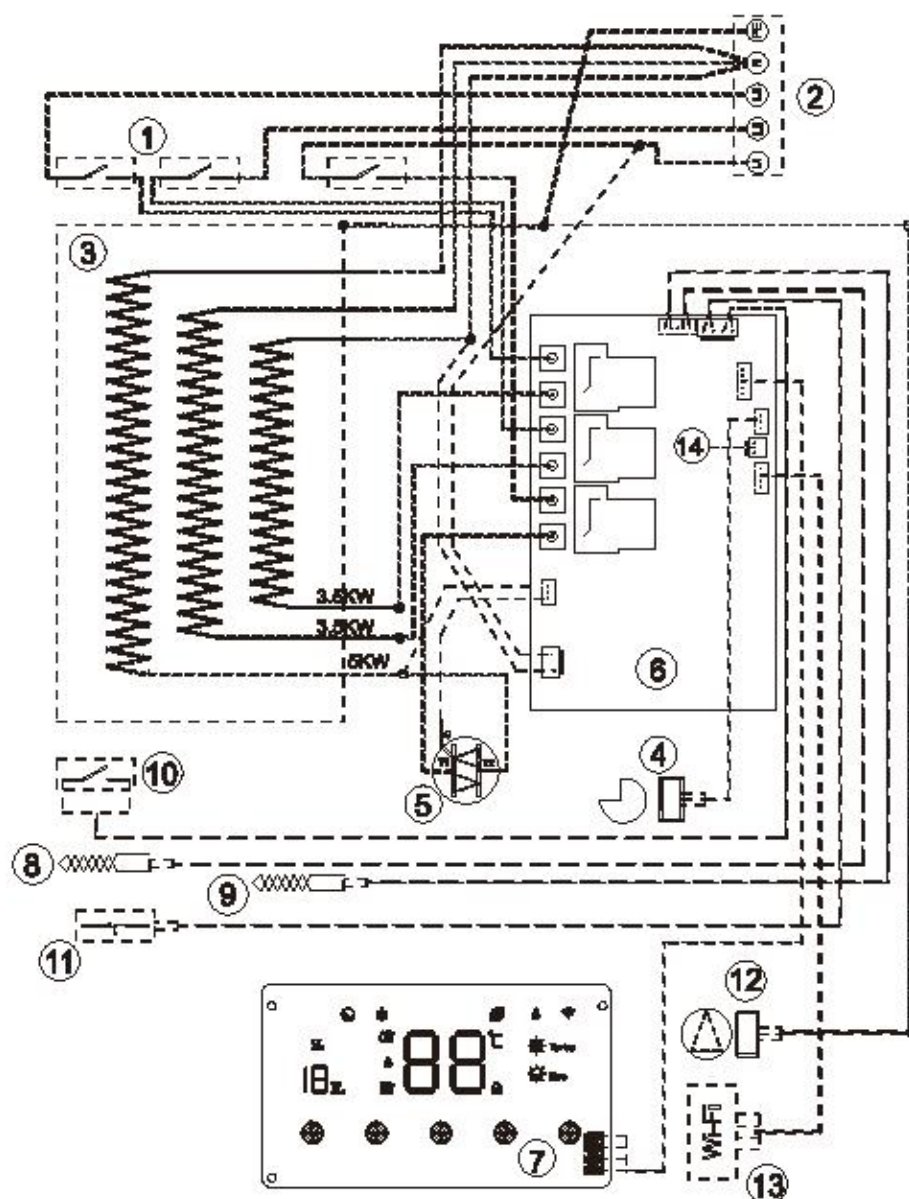
Рис. 15. Электрическая схема THERMEX Grizzly 5-12 Wi-Fi
