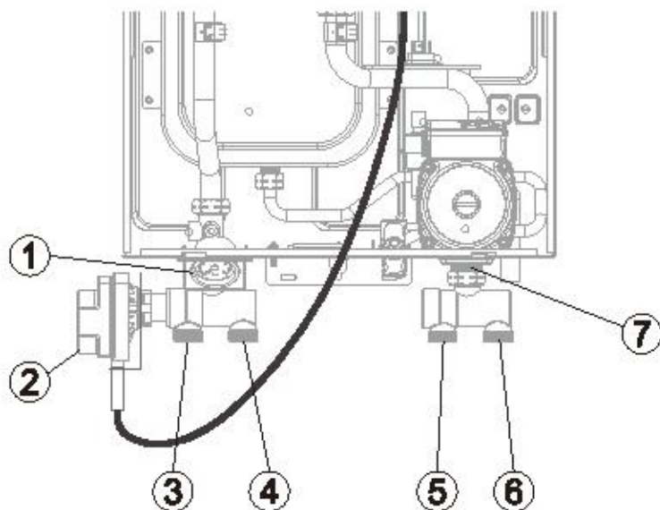
Рис. 15. Присоединение трехходового клапана
