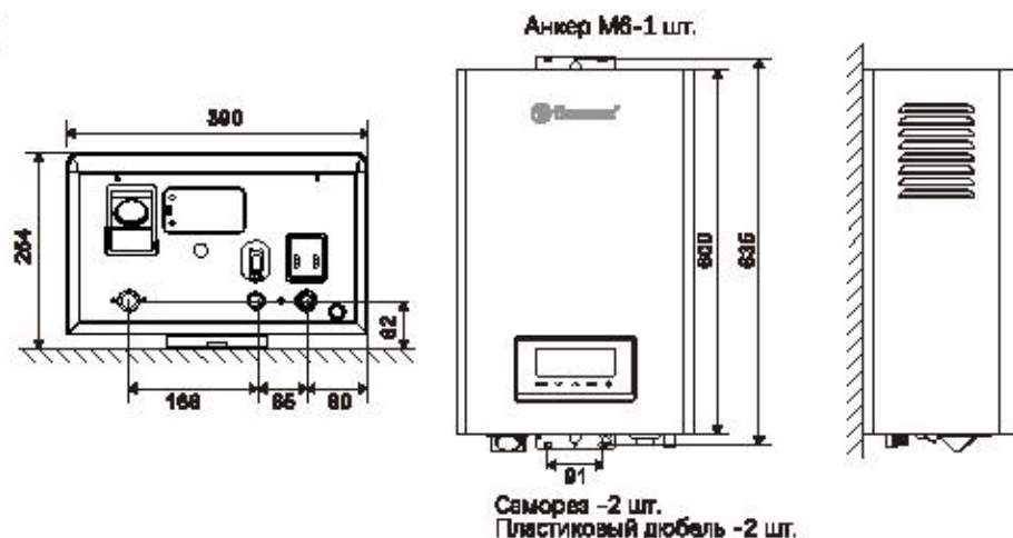
Рис. 6. Монтажные размеры
