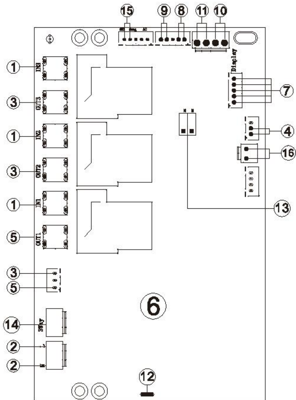
Рис. 20. Электрическая схема основной платы управления
