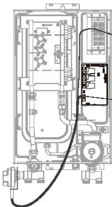
Рис. 16. Подключение трехходового клапана
