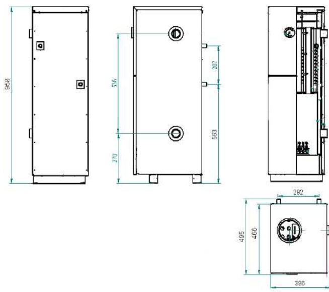
рис. 3 Аппараты АОГВ/АОГБК -17,4-1; АОГВ/АОГБК -17,4Т-1.
