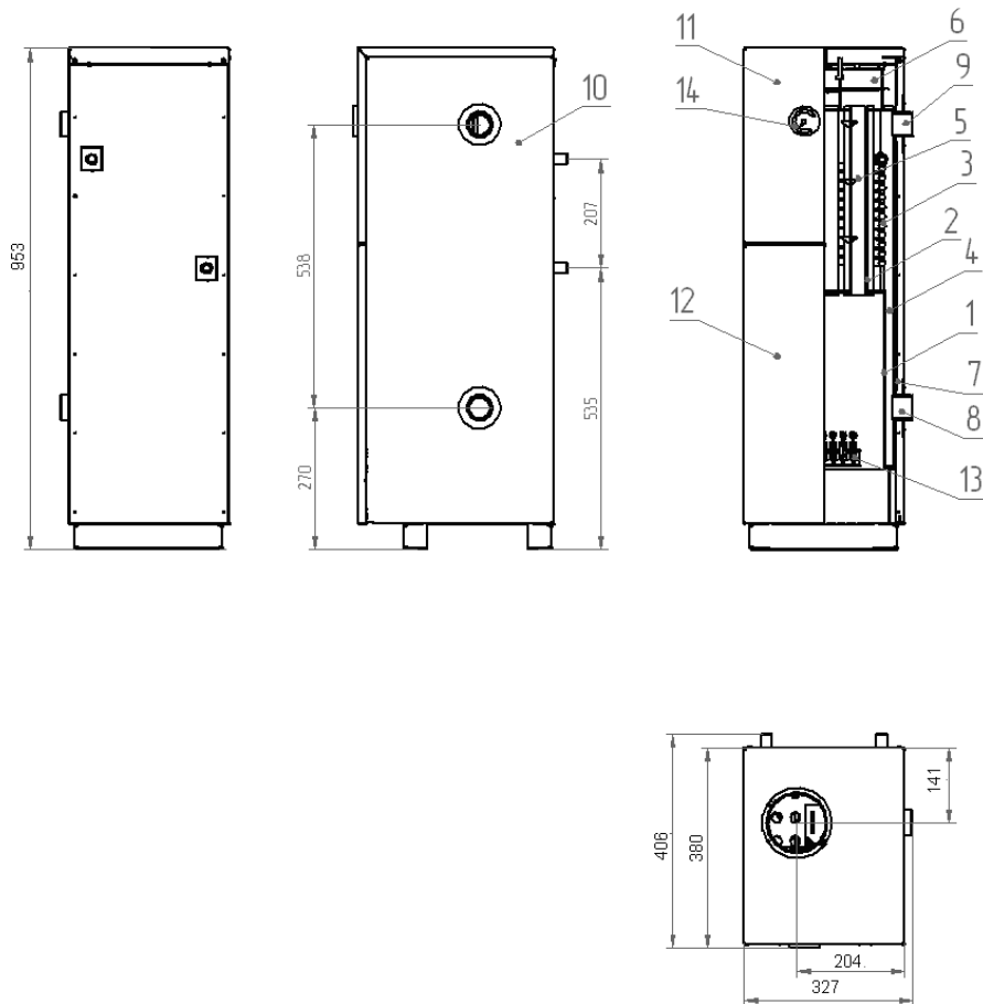
рис.1 Аппараты АОВГ/АОВГК -11,6-1; АОВГ/АОВГК -11,6Т-1
