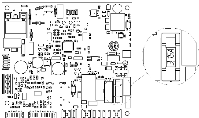
Рис. 11. Расположение предохранителя
