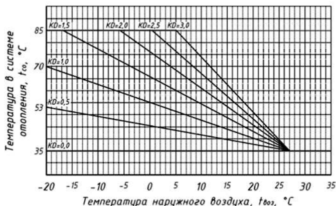
Рис. 9. Кривые нагрева
