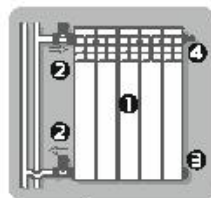
Байпасное (двухтрубная система отопления)
