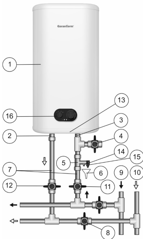
Рисунок 1. Схема подключения ЭВН к водопроводу сверху и снизу
