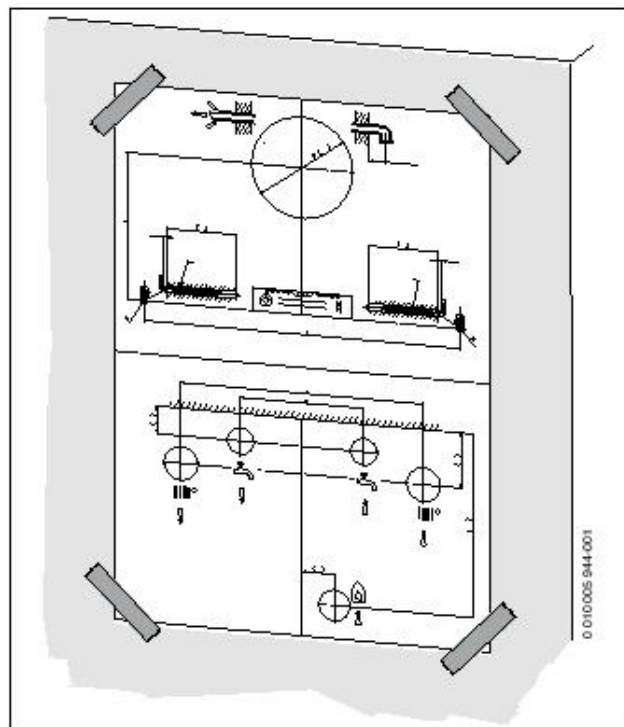
Рис. 12 Монтажный шаблон
