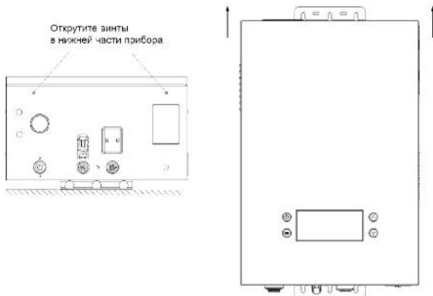
Рис. 7. Демонтаж лицевой панели
