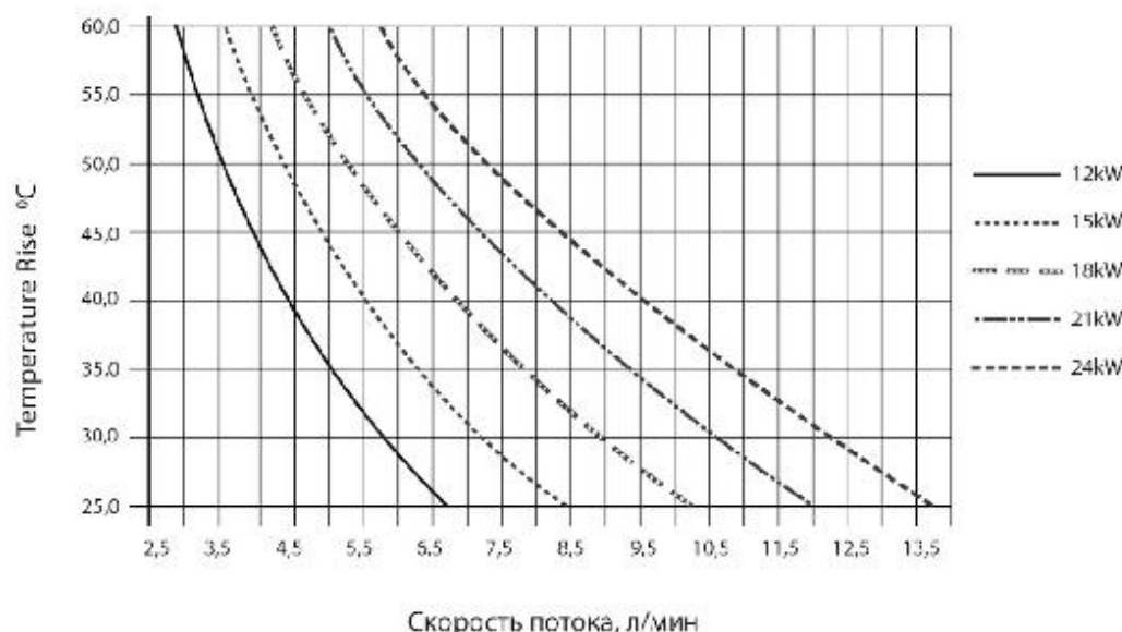
Рис. 4. График производительности системы ГВС
