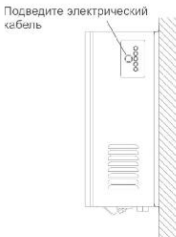
Рис. 8. Расположение панели вывода электрического кабеля
