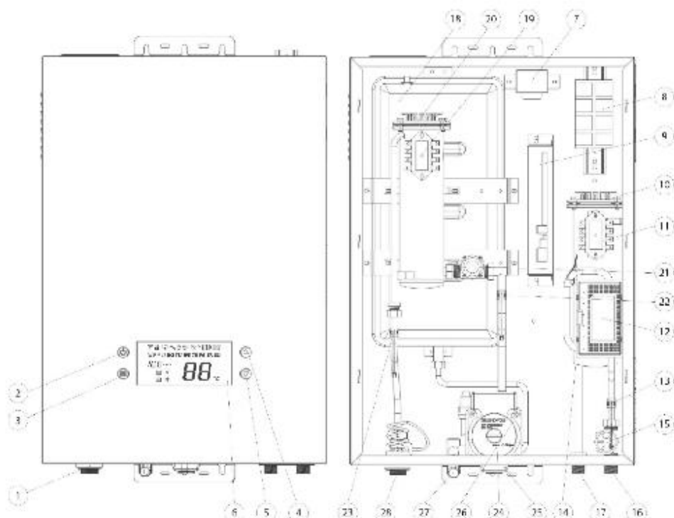
Рис. 1. Конструкция изделия
