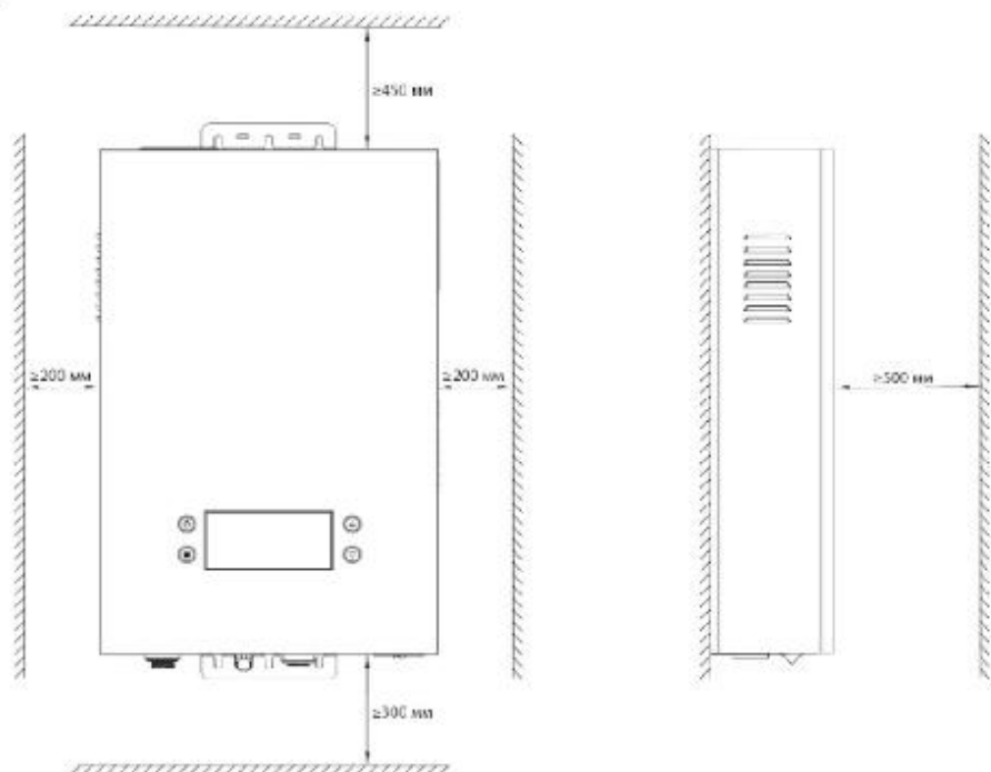
Рис. 5. Минимальные расстояния от электрического котла до поверхностей.
