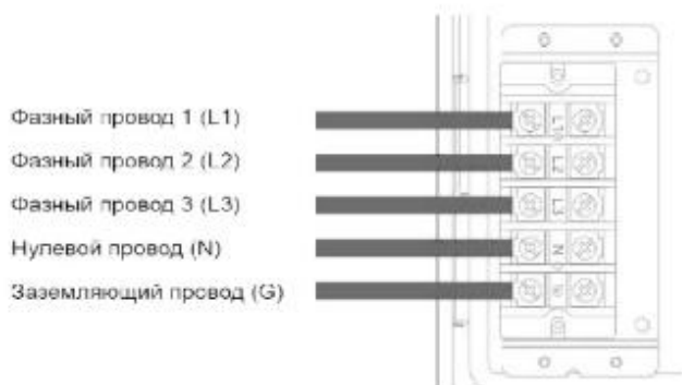
Рис.9. Подключение прибора
