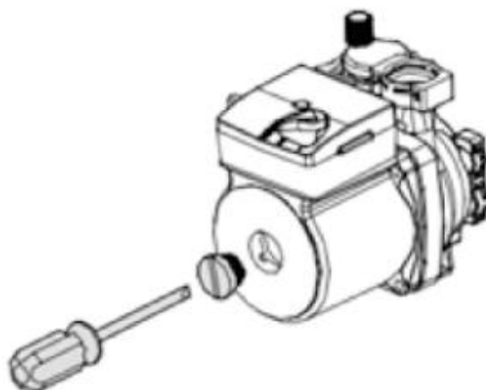
Рис.15. Проверка насоса
