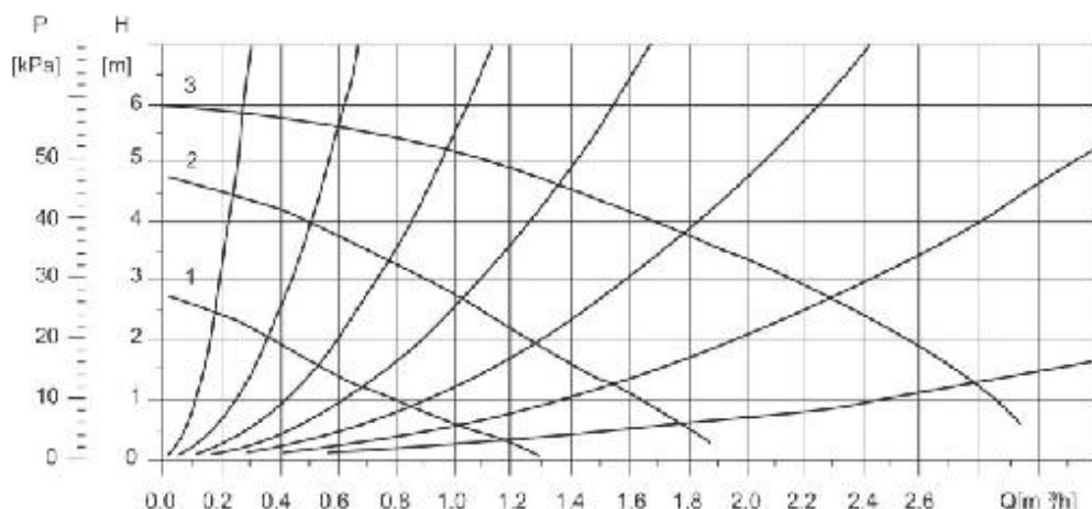
Рис. 12. Кривая характеристик давления насоса
