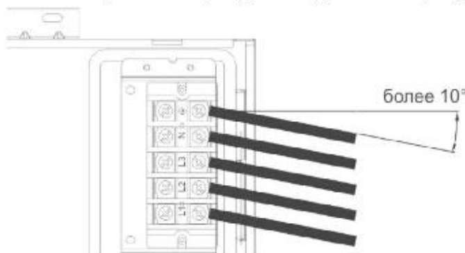
Рис. 10. Расположение сетевого кабеля
