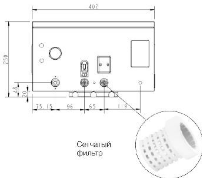
Рис. 13. Сетчатый фильтр
