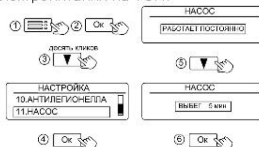
Рисунок 26. Настройка времени выбега циркуляционного насоса
