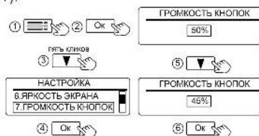
Рисунок 21. Настройка громкости кнопок
