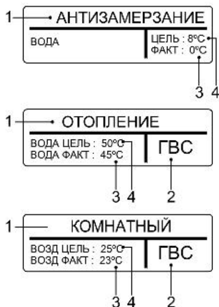
Рисунок 4. Виды главного окна
