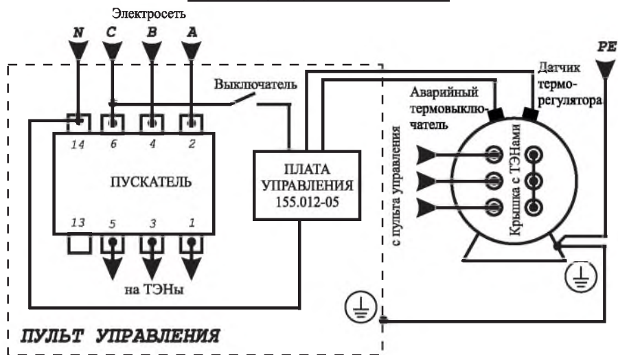
Рисунок 6. Электрическая схема подключения
