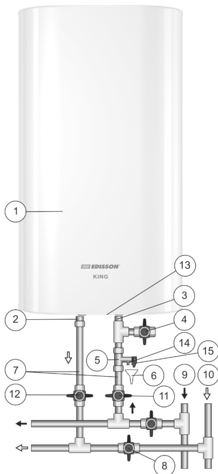
Рисунок 1. Схема подключения ЭВН к водопроводу сверху и снизу
