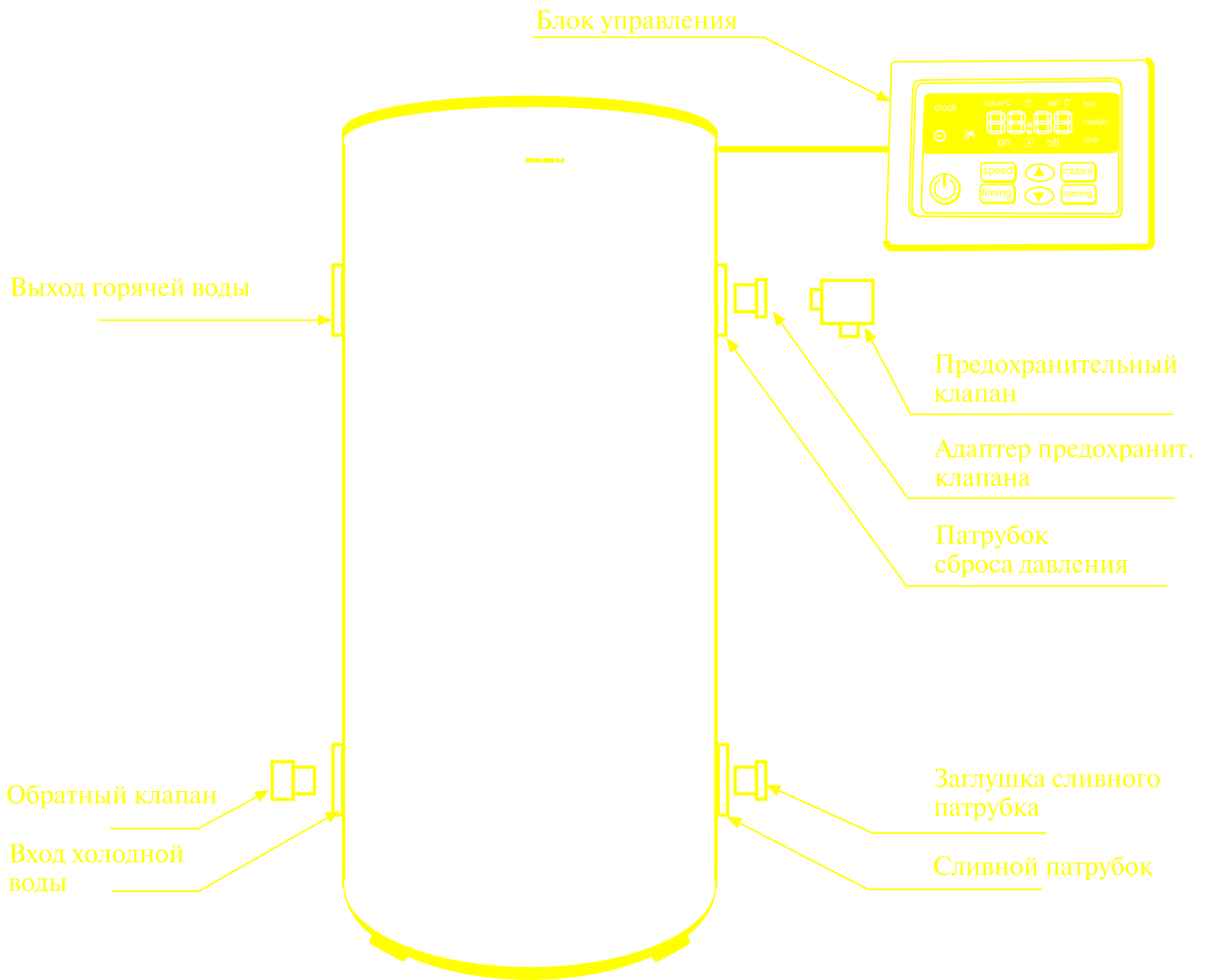
Рис. 3. Схема подключений.
